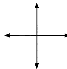
17 座標軸
