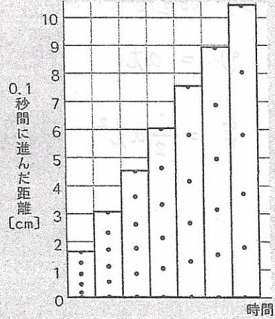
(b) 斜面の角度が大きいとき(約9°)
