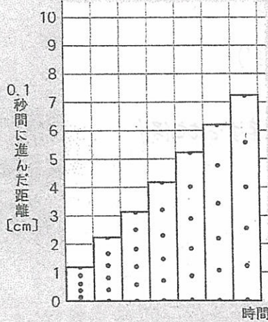
(a) 斜面の角度が小さいとき(約6°)
